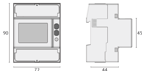
Abmessungen (mm):
