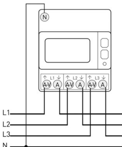
3 Phasen - 4 Leiter
